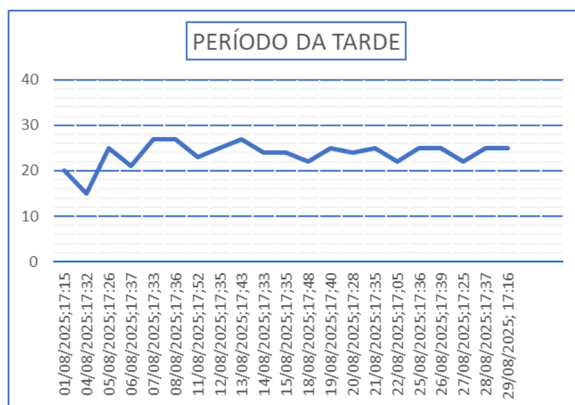
Gráfico 34 – Monitoramento de pressão PCP - 16.
