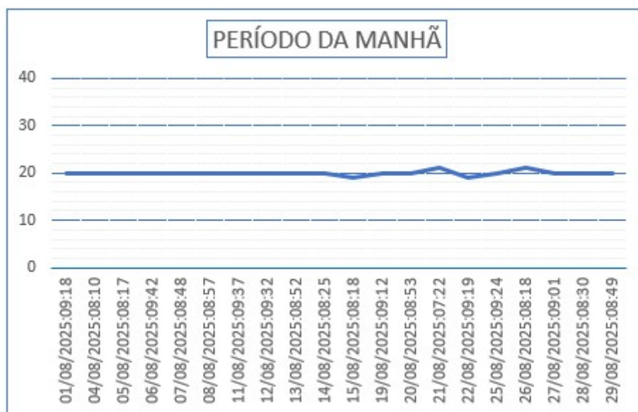
Gráfico 15 - Monitoramento de Pressão do PCP 07.
