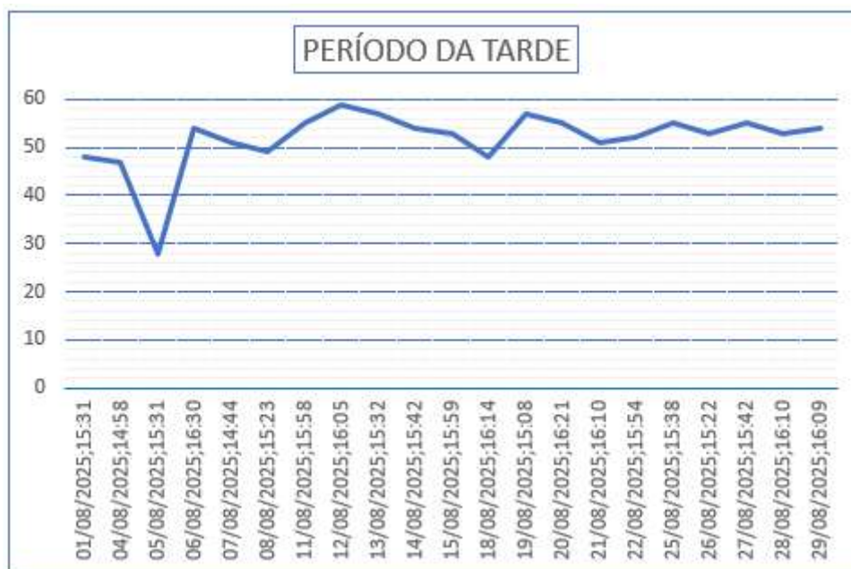
Gráfico 26 - Monitoramento de Pressão do PCP 12.
