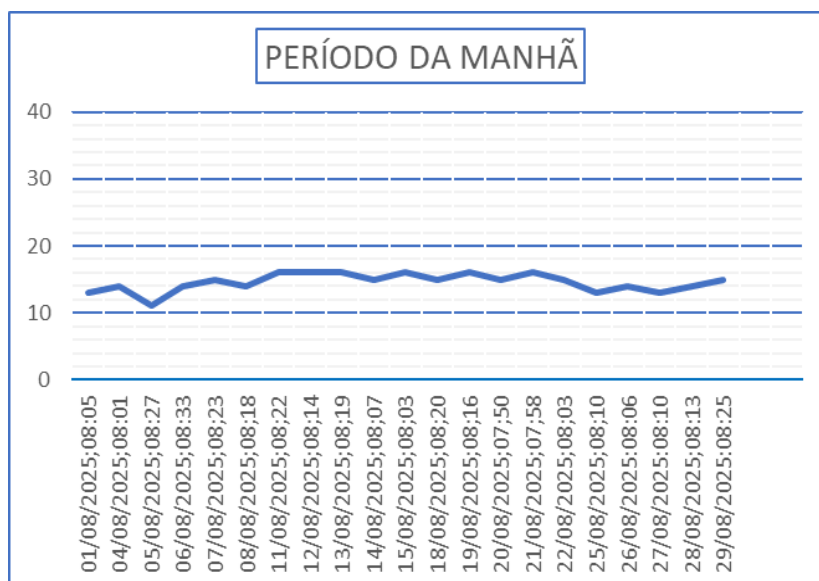
Gráfico 05 – Monitoramento de Pressão do PCP -02.
