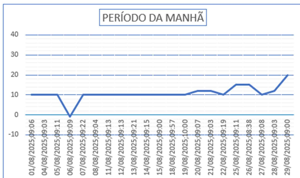
Gráfico 09 – Monitoramento de Pressão do PCP 04.
