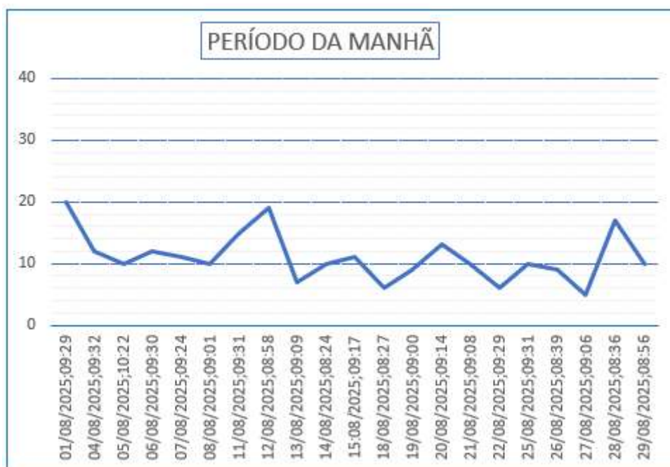
Gráfico 27 – Monitoramento de Pressão do PCP 13.
