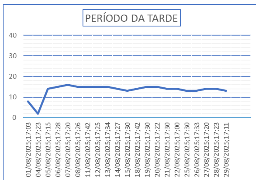
Gráfico 28 – Monitoramento de pressão PCP - 13.
