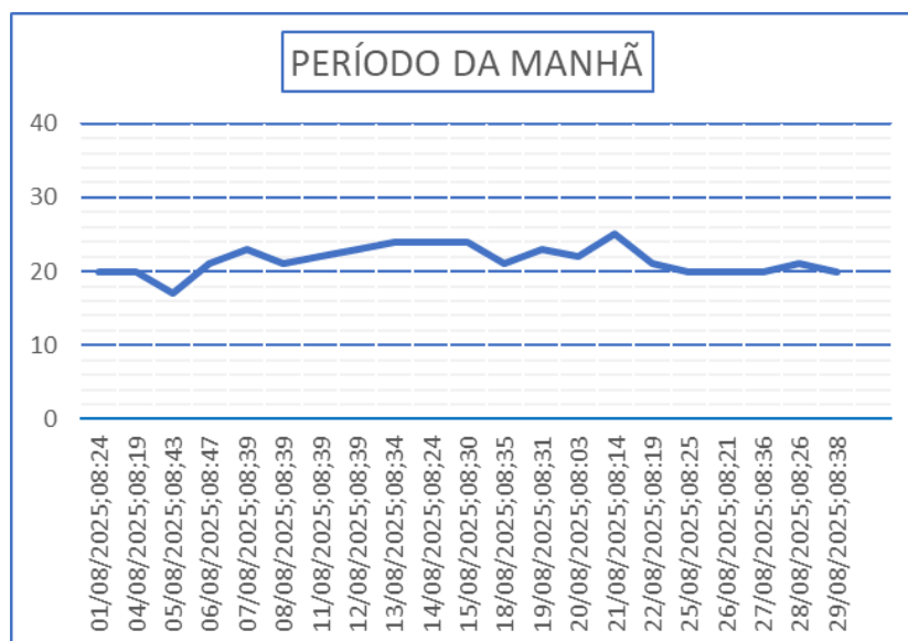
Gráfico 09 – Monitoramento de Pressão do PCP -04.
