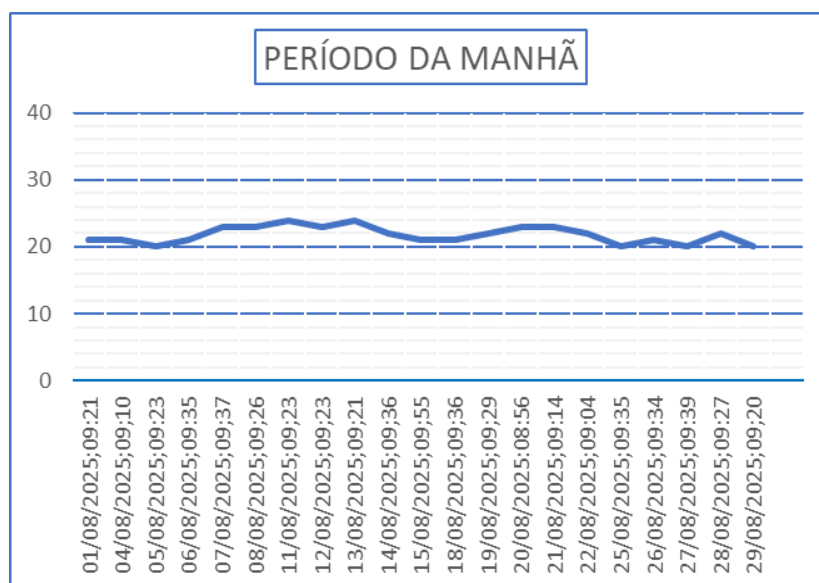
Gráfico 21 – Monitoramento de pressão PCP - 10.
