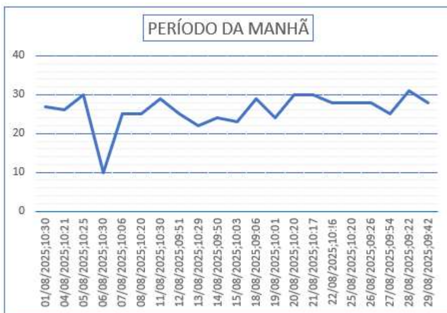
Gráfico 45 – Monitoramento de Pressão do PCP 22.
