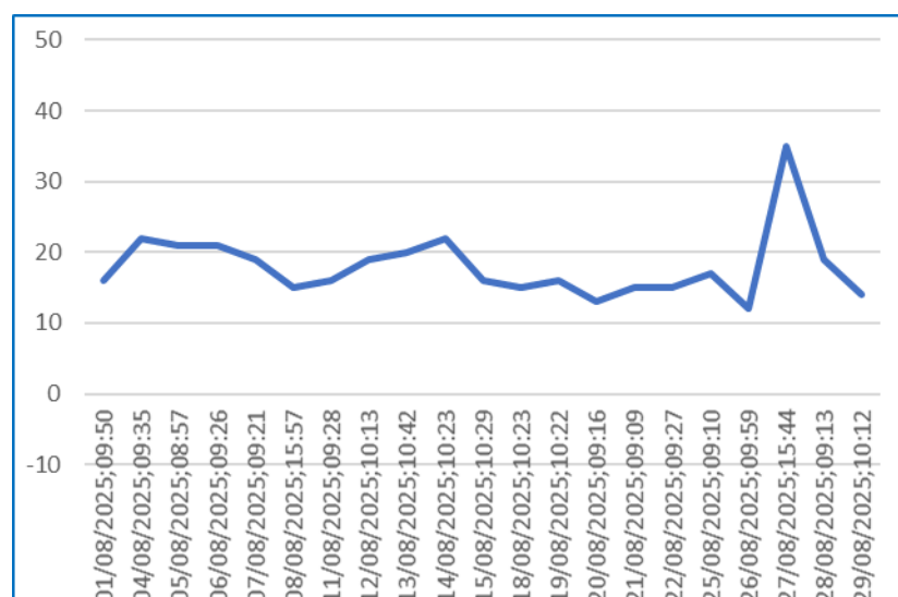
Gráfico 13 – Monitoramento de Pressão PCP -12.
