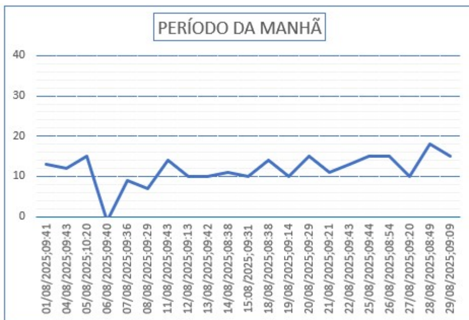
Gráfico 31 – Monitoramento de Pressão do PCP 15.
