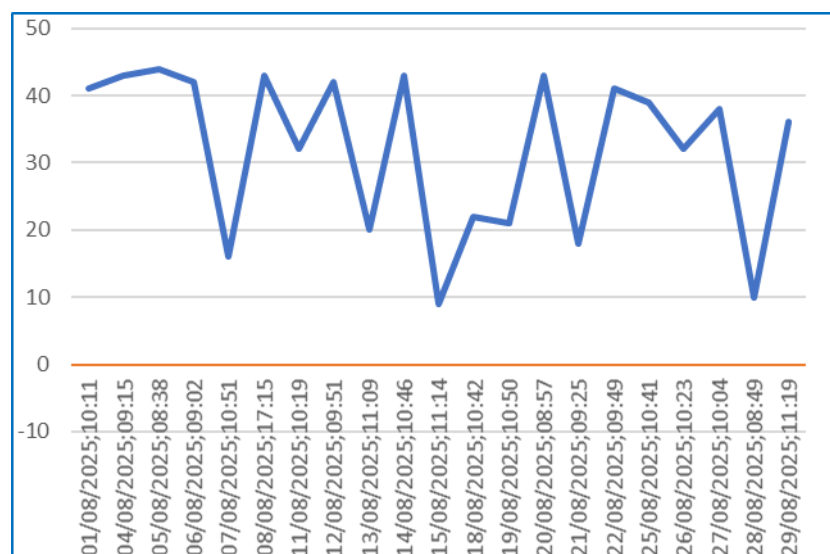
Gráfico 19 – Monitoramento de pressão PCP - 18.
