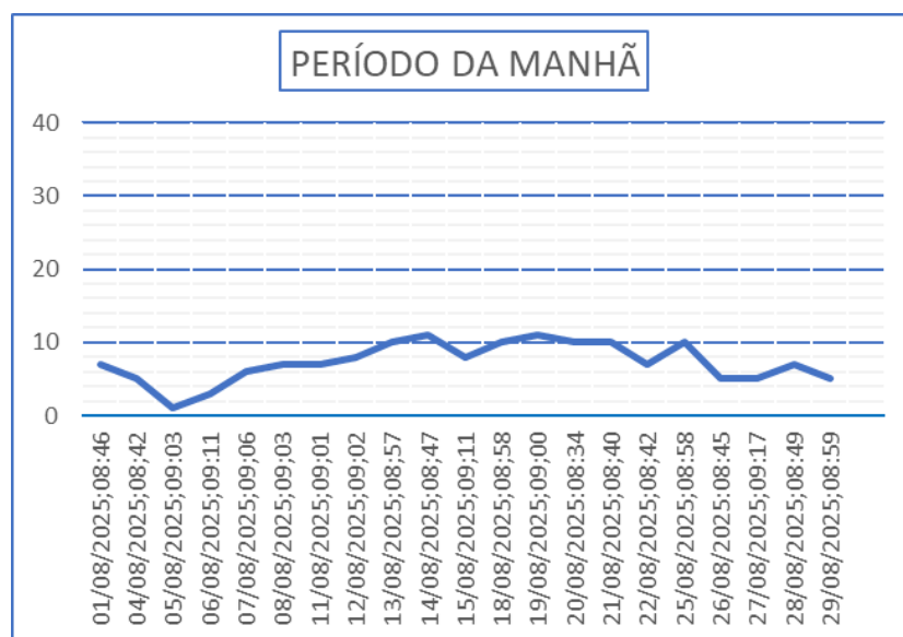
Gráfico 15 – Monitoramento de Pressão PCP -07.
