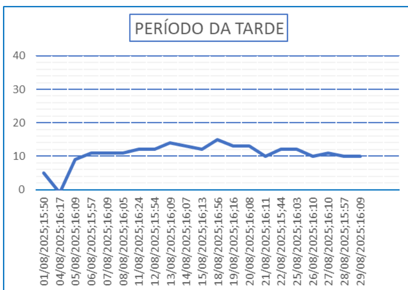
Gráfico 06 – Monitoramento de Pressão do PCP -02.
