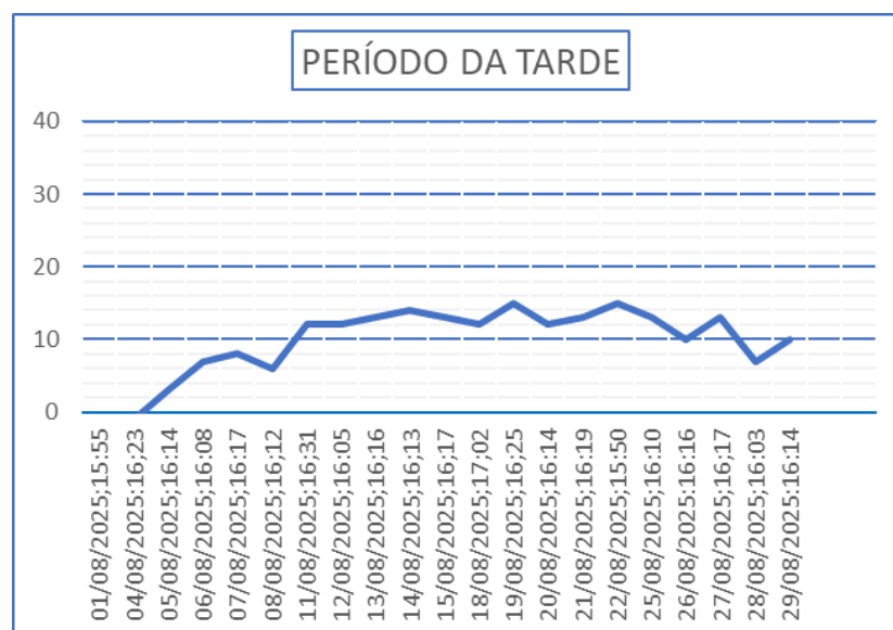
Gráfico 08– Monitoramento de Pressão do PCP -03.
