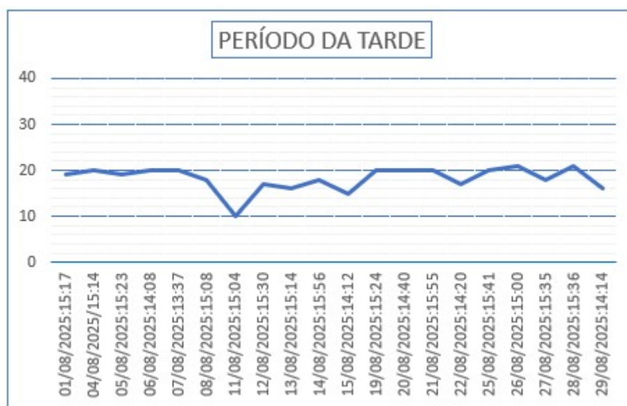
Gráfico 14 - Monitoramento de Pressão do PCP 06.
