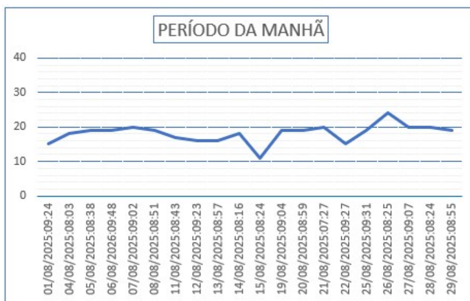
Gráfico 13 - Monitoramento de Pressão do PCP 06.
