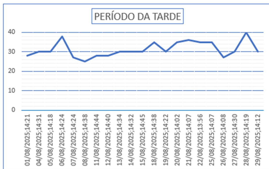
Gráfico 04 – Monitoramento de Pressão do PCP 01.
