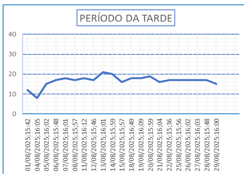
Gráfico 04 – Monitoramento de Pressão do PCP -01.
