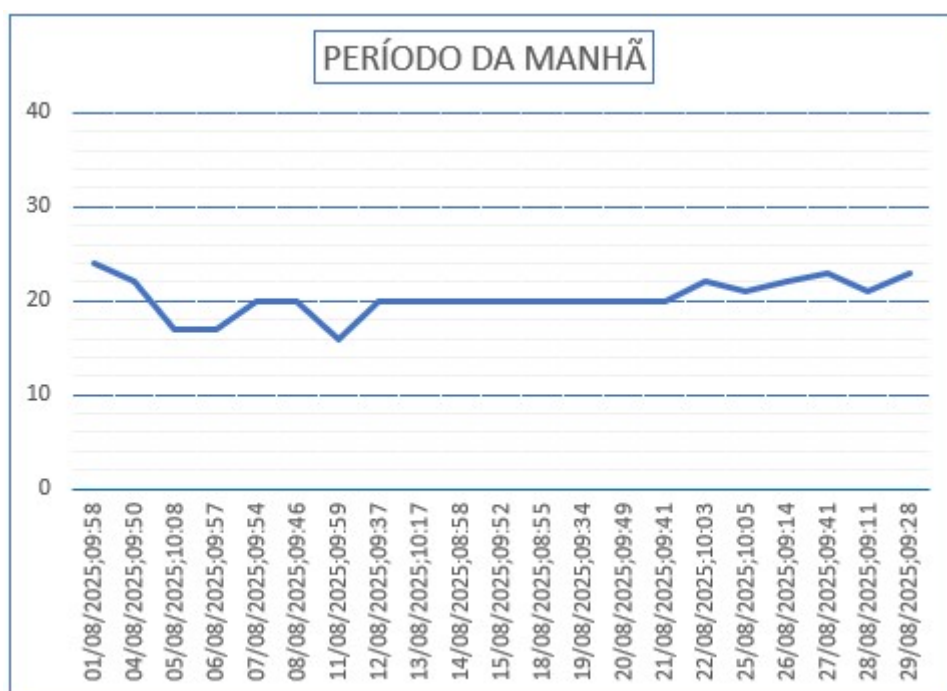
Gráfico 39 – Monitoramento de Pressão do PCP 19.
