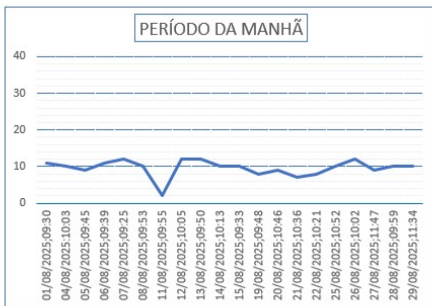
Gráfico 11 - Monitoramento de Pressão do PCP 05.
