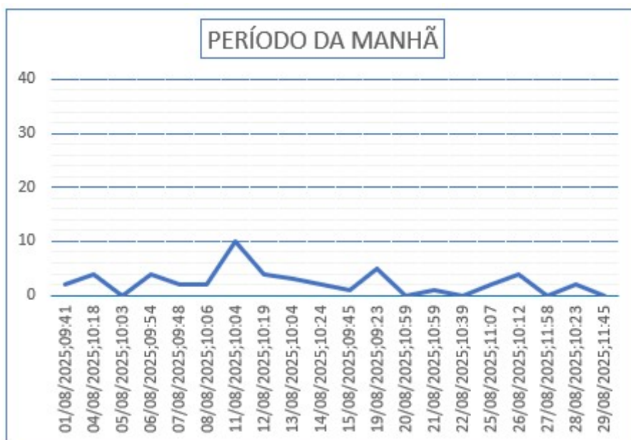
Gráfico 13 - Monitoramento de Pressão do PCP 06.
