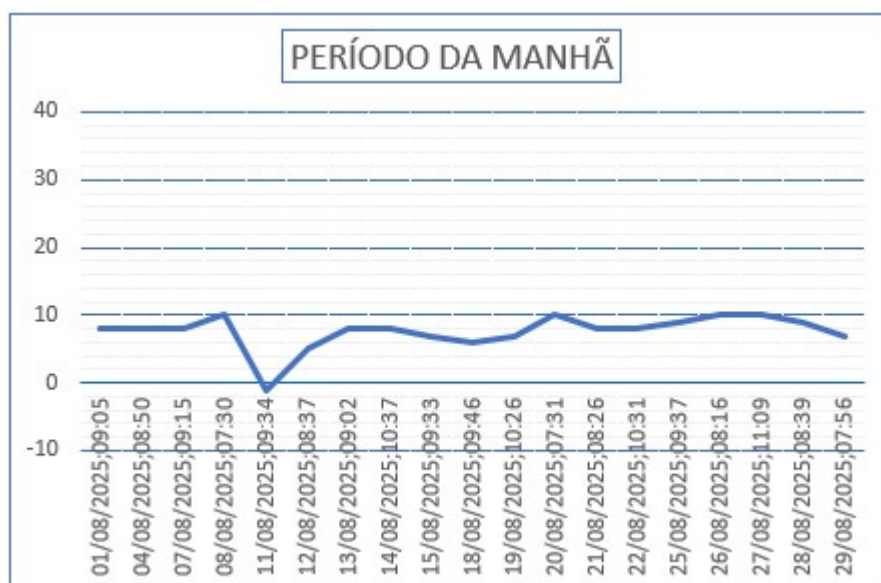
Gráfico 17 - Monitoramento de Pressão do PCP 08.
