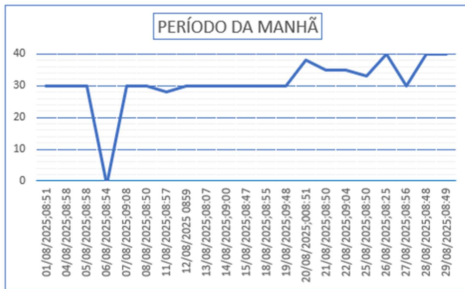
Gráfico 03 – Monitoramento de Pressão do PCP 01.
