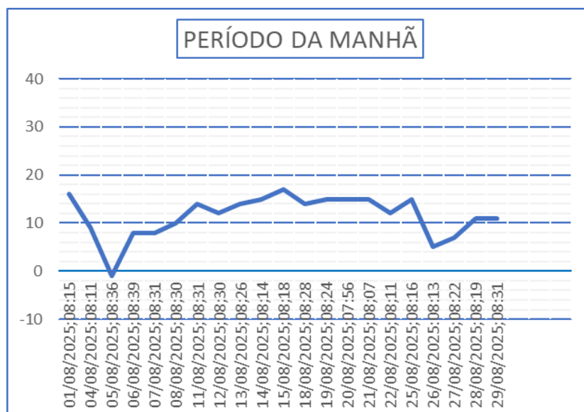
Gráfico 07 – Monitoramento de Pressão do PCP -03.
