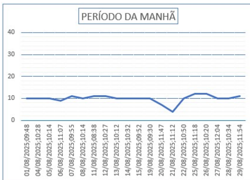
Gráfico 15 - Monitoramento de Pressão do PCP 07.
