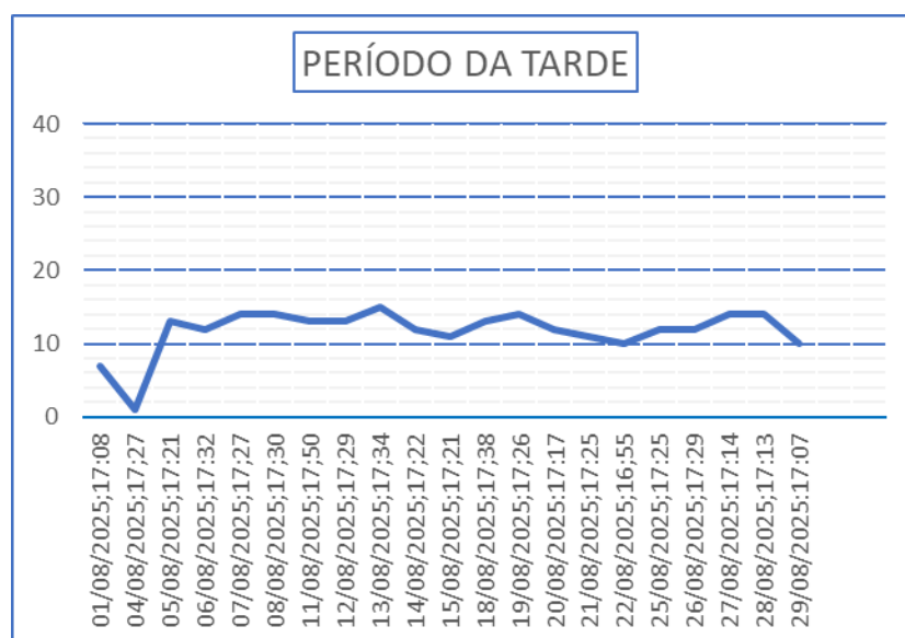
Gráfico 26 – Monitoramento de pressão PCP - 12.
