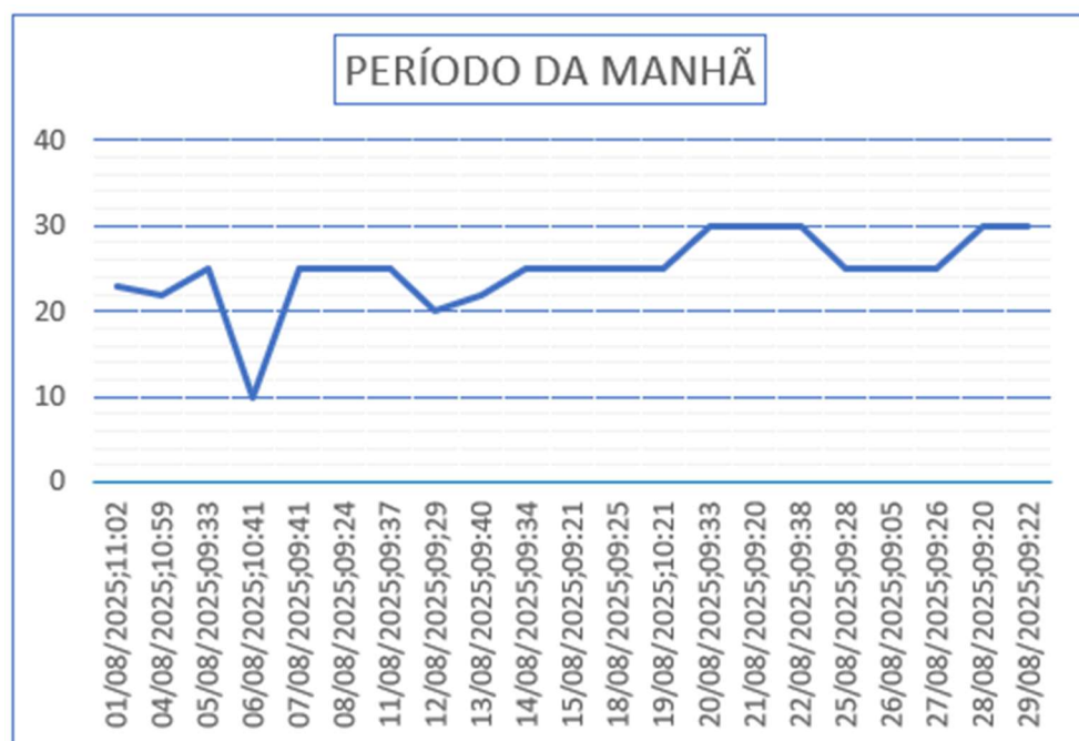
Gráfico 17 – Monitoramento de Pressão do PCP 08.
