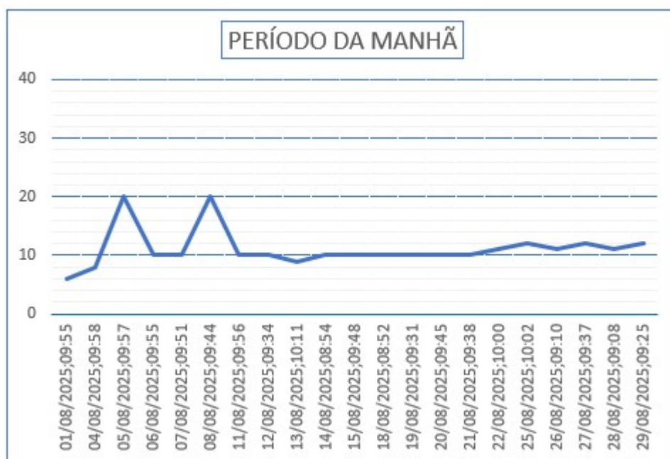
Gráfico 37 – Monitoramento de Pressão do PCP 18.
