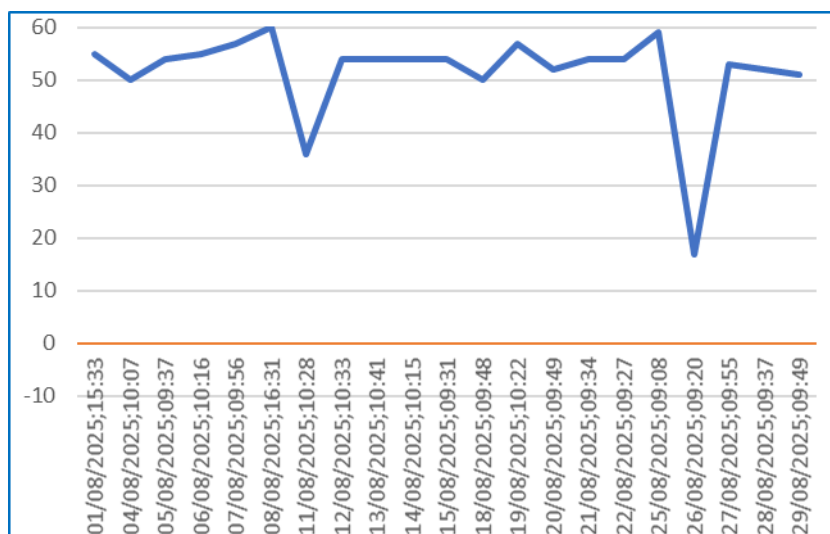
Gráfico 08 – Monitoramento de Pressão do PCP -07.
