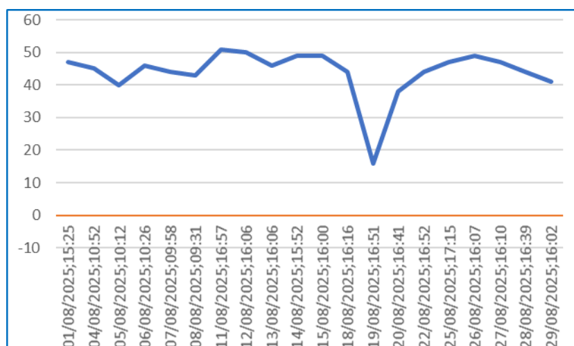
Gráfico 30 – Monitoramento de pressão PCP - 29.
