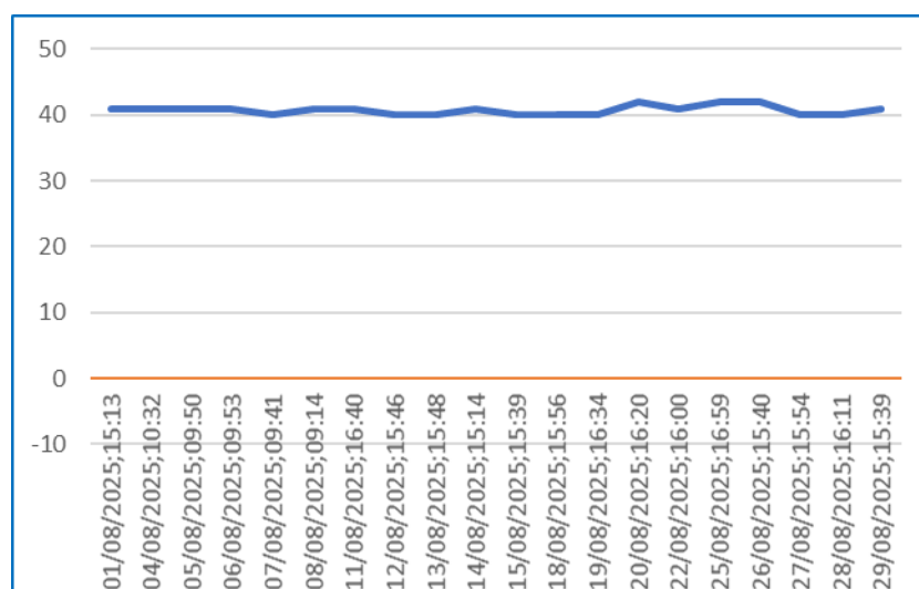
Gráfico 22 – Monitoramento de pressão PCP - 21.
