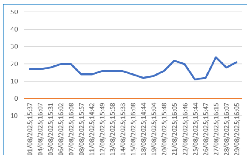
Gráfico 32 – Monitoramento de pressão PCP - 31.
