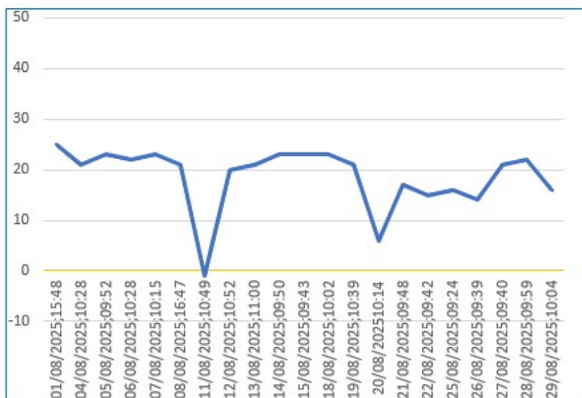
Gráfico 02 – Monitoramento de Pressão do PCP - 01.
