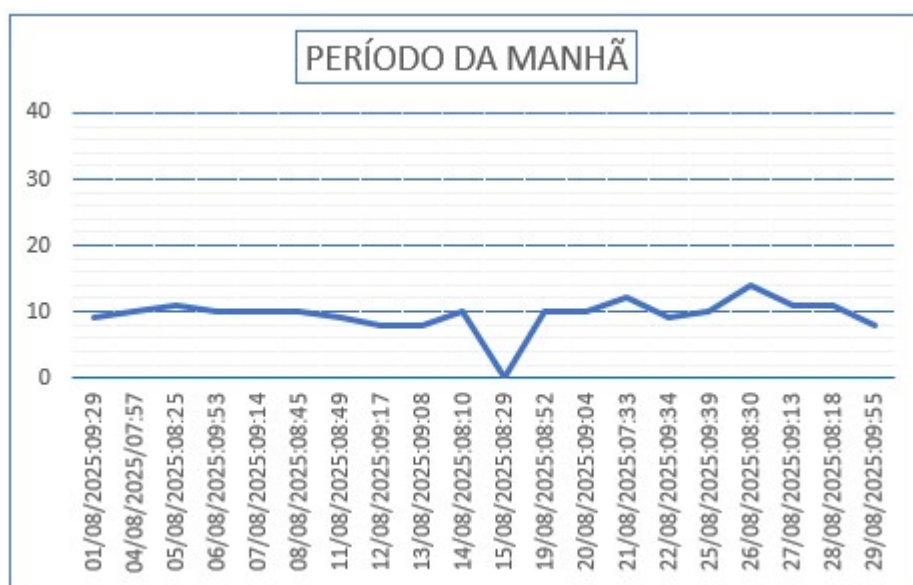
Gráfico 09 – Monitoramento de Pressão do PCP 04.
