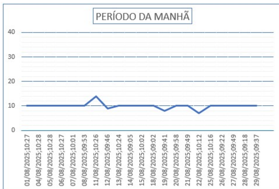
Gráfico 43 – Monitoramento de Pressão do PCP 21.
