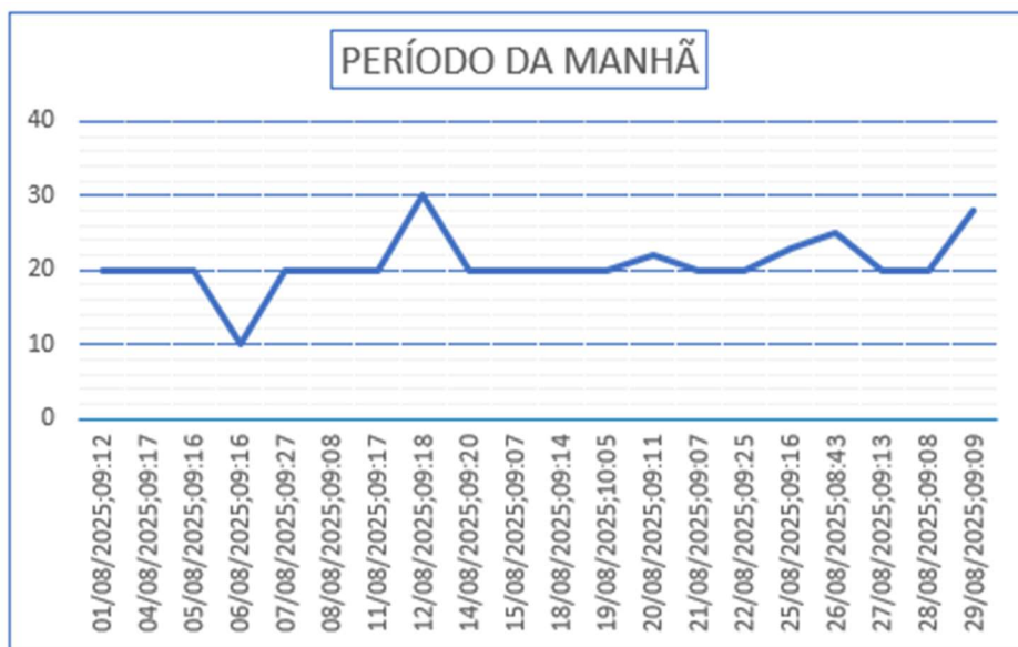
Gráfico 11 – Monitoramento de Pressão do PCP 05.
