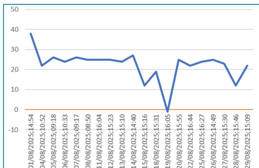
Gráfico 27 – Monitoramento de pressão PCP - 26.
