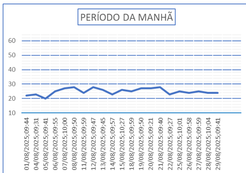
Gráfico 33 – Monitoramento de pressão PCP - 16.
