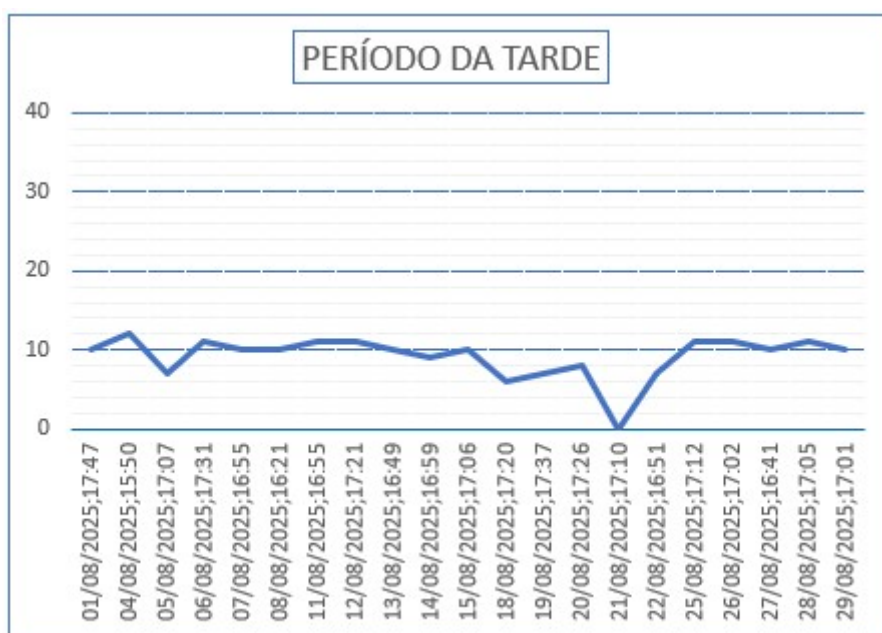
Gráfico 16 - Monitoramento de Pressão do PCP 07.
