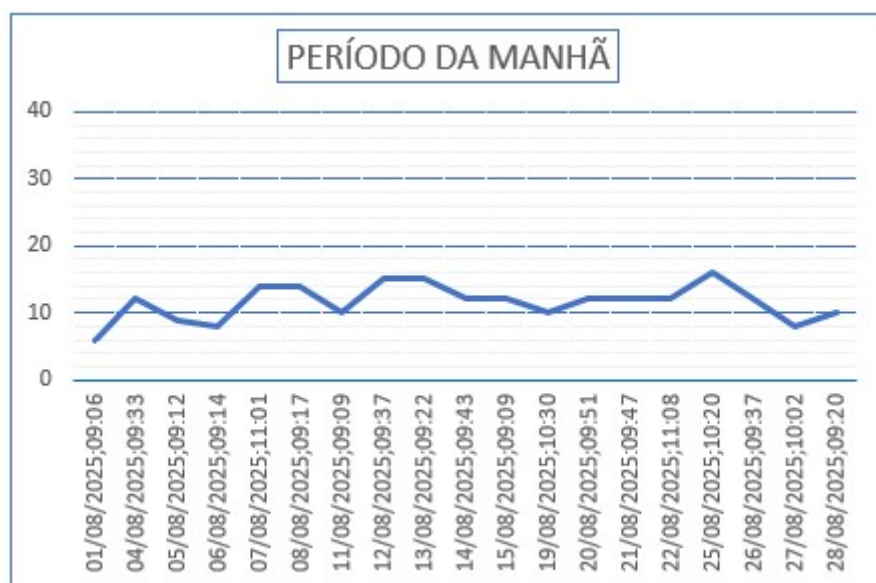
Gráfico 05 – Monitoramento de Pressão do PCP 02.
