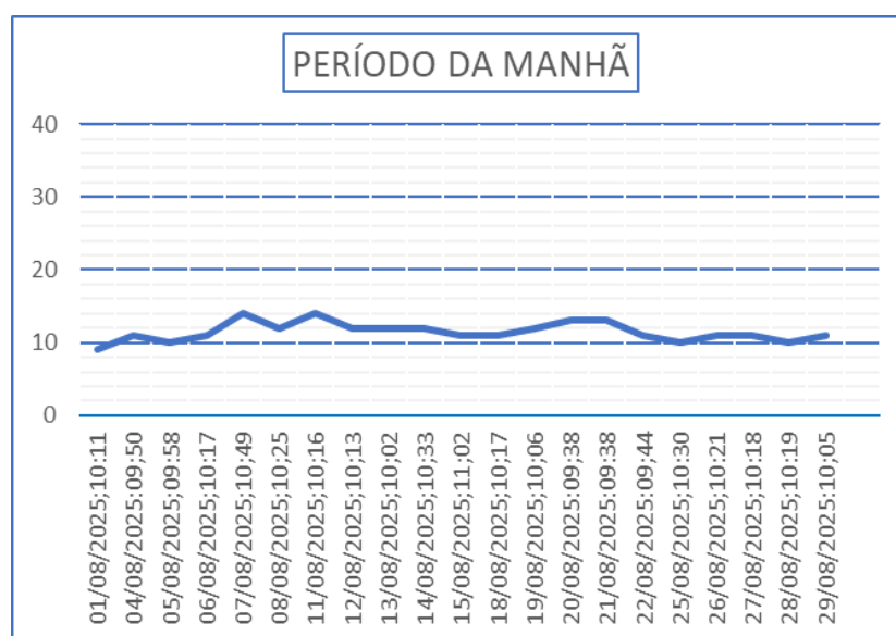
Gráfico 31 – Monitoramento de pressão PCP - 15.
