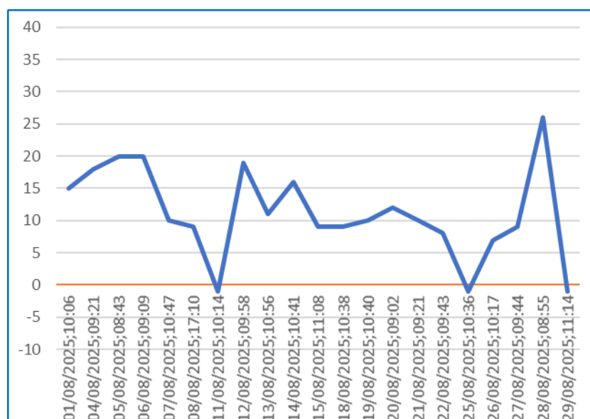
Gráfico 18 – Monitoramento de pressão PCP - 17.
