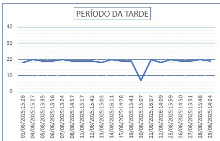
Gráfico 12 - Monitoramento de Pressão do PCP 05.
