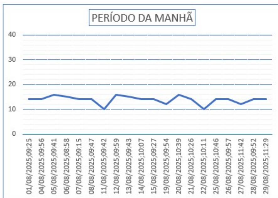
Gráfico 09 – Monitoramento de Pressão do PCP 04.
