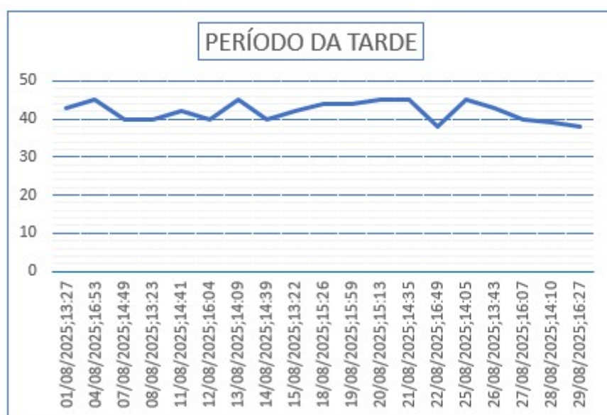
Gráfico 14 - Monitoramento de Pressão do PCP 06.
