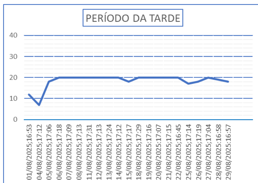
Gráfico 22 – Monitoramento de pressão PCP - 10.
