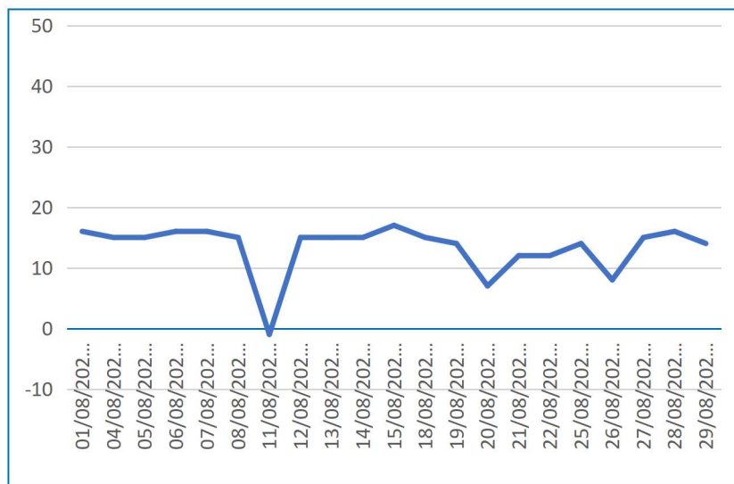
Gráfico 04 – Monitoramento de Pressão do PCP -03.
