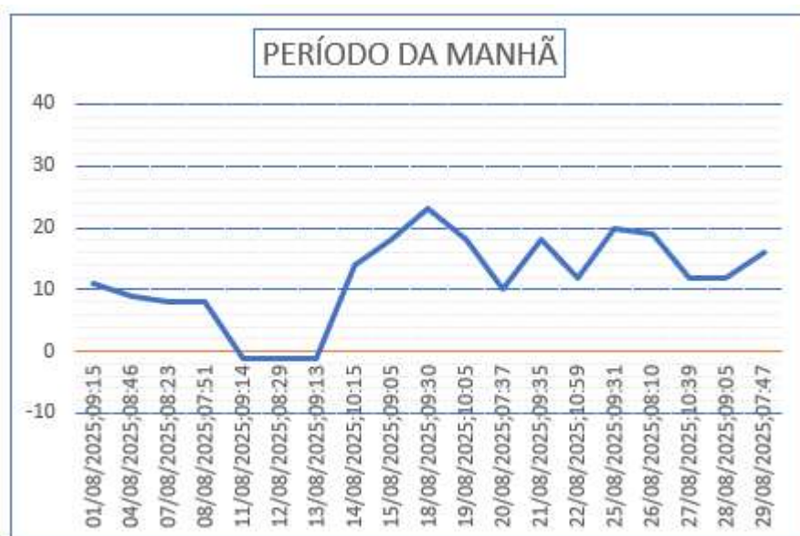
Gráfico 09 – Monitoramento de Pressão do PCP 04.
