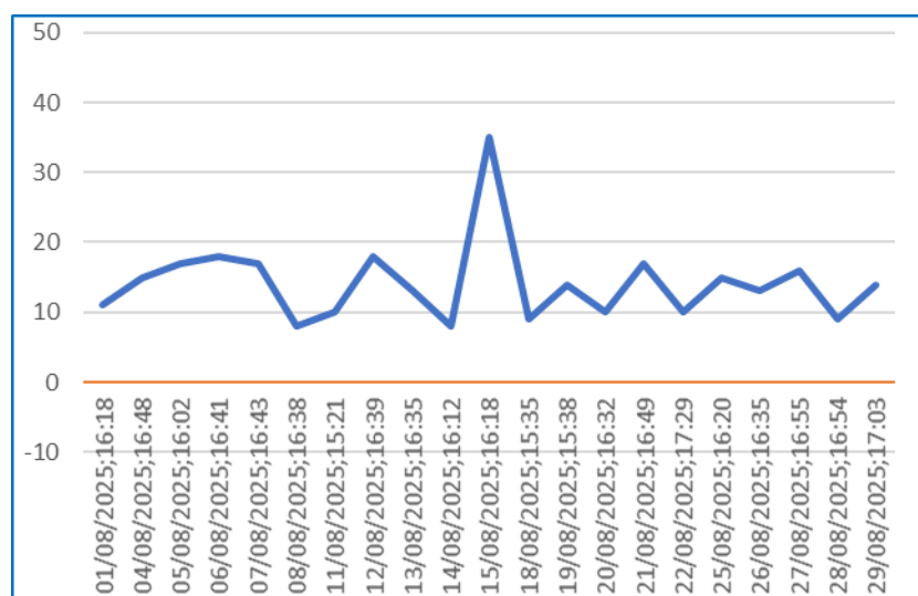
Gráfico 36 – Monitoramento de pressão PCP - 35.
