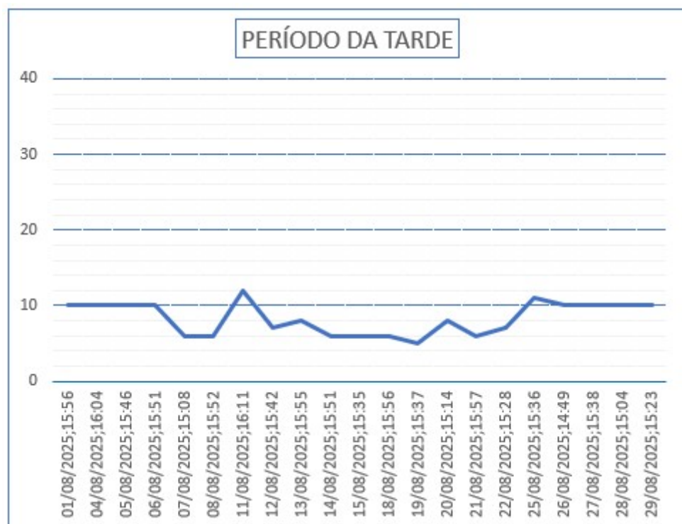
Gráfico 44 – Monitoramento de Pressão do PCP 21.
