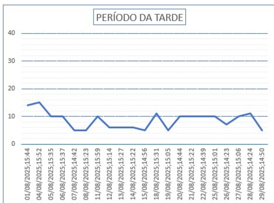
Gráfico 30 – Monitoramento de Pressão do PCP 14.
