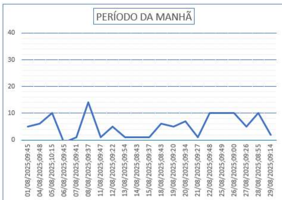
Gráfico 33 – Monitoramento de Pressão do PCP 16.
