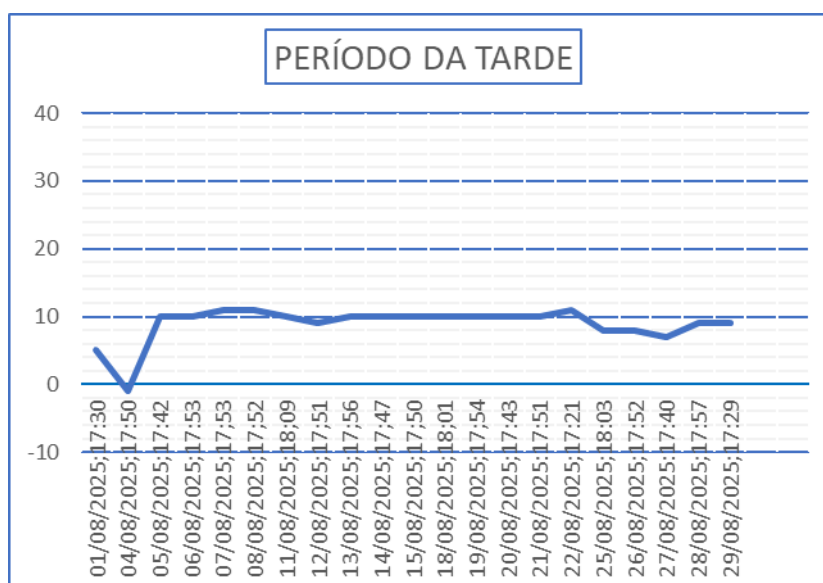
Gráfico 32 – Monitoramento de pressão PCP - 15.
