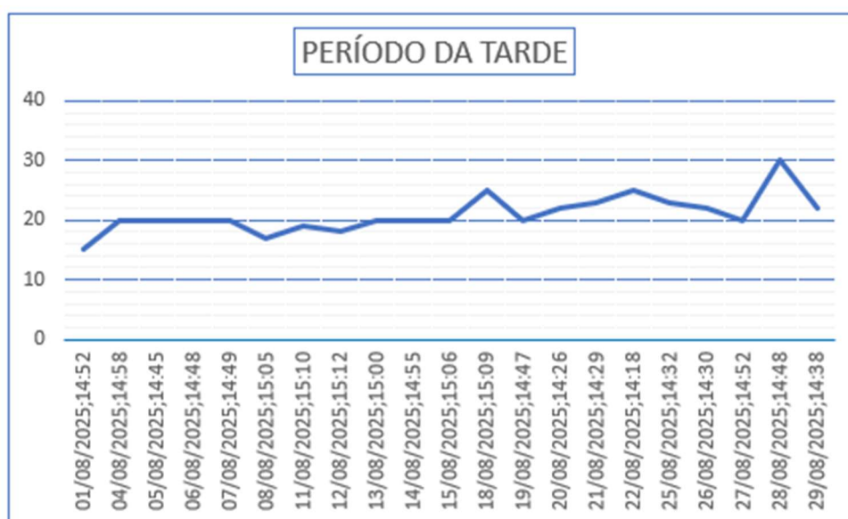
Gráfico 16 – Monitoramento de Pressão do PCP 07.
