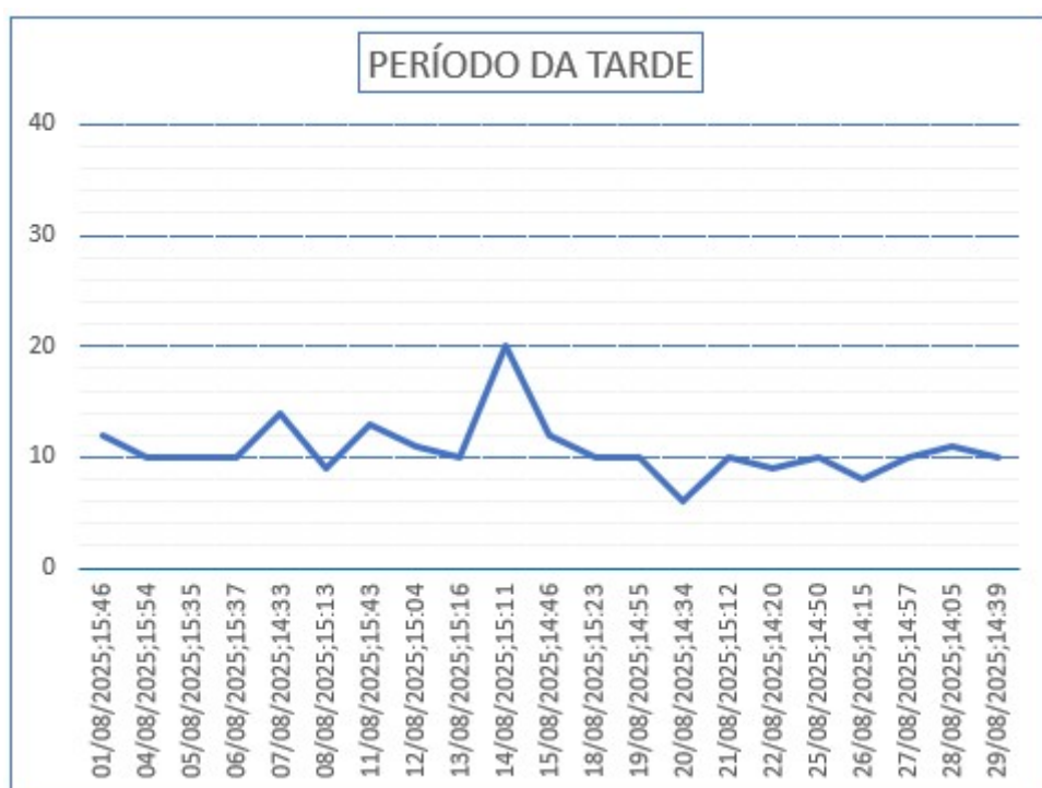
Gráfico 28 – Monitoramento de Pressão do PCP 13.
