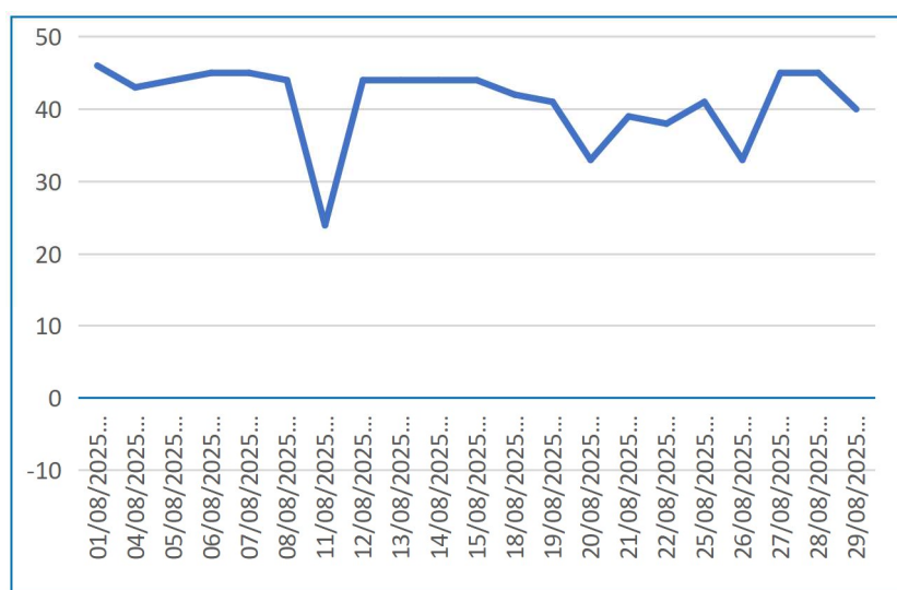
Gráfico 05 – Monitoramento de Pressão do PCP -04.
