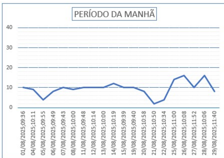
Gráfico 19 - Monitoramento de Pressão do PCP 09.
