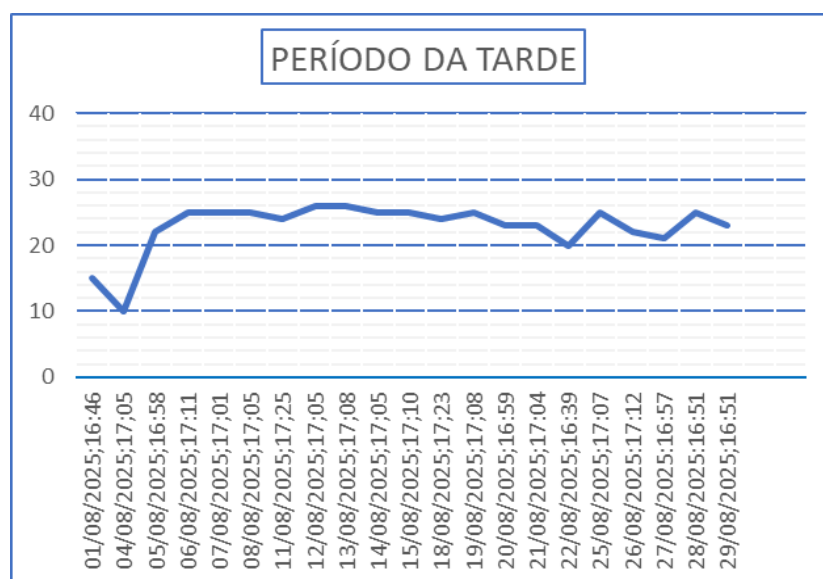
Gráfico 20 – Monitoramento de pressão PCP - 09.
