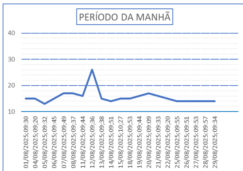
Gráfico 27 – Monitoramento de pressão PCP - 13.
