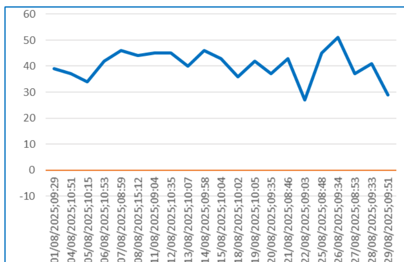
Gráfico 21 – Monitoramento de pressão PCP - 20.
