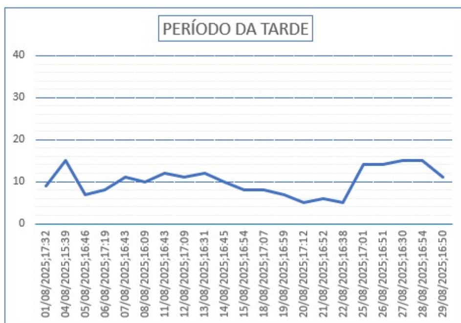
Gráfico 20 - Monitoramento de Pressão do PCP 09.
