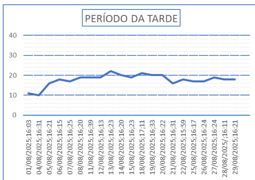
Gráfico 10 – Monitoramento de Pressão do PCP -04.
