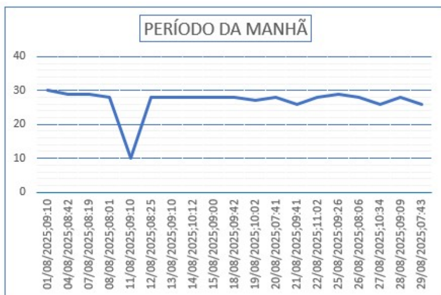
Gráfico 11 - Monitoramento de Pressão do PCP 05.
