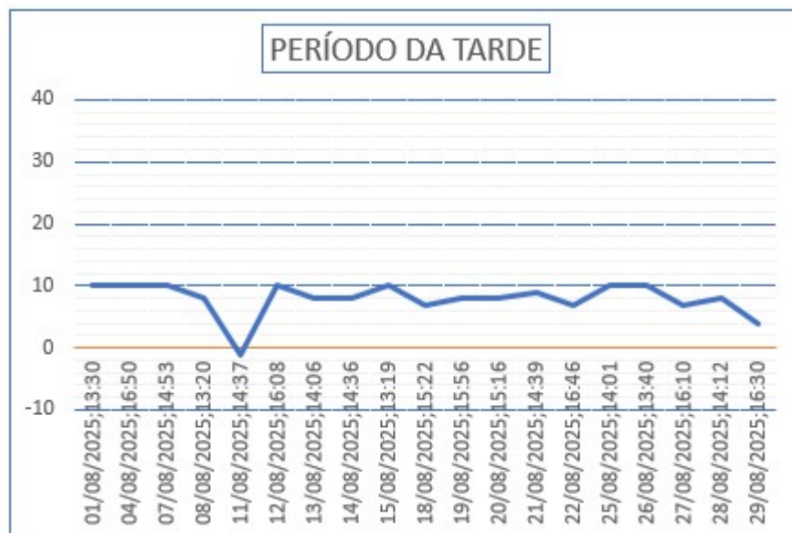
Gráfico 06 – Monitoramento de Pressão do PCP 02.
