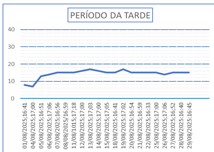
Gráfico 18 – Monitoramento de pressão PCP - 08.
