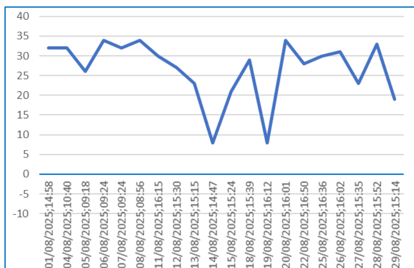
Gráfico 26 – Monitoramento de pressão PCP - 25.
