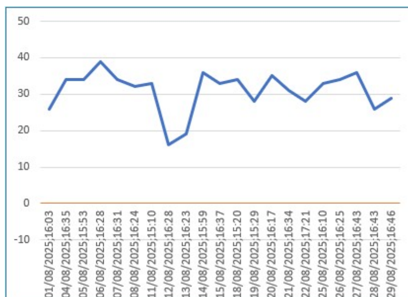
Gráfico 41 – Monitoramento de pressão PCP - 40.
