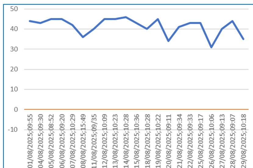
Gráfico 14 – Monitoramento de Pressão PCP -13.
