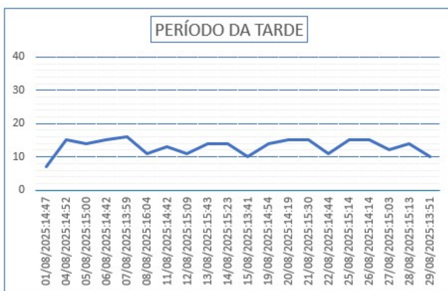
Gráfico 06 – Monitoramento de Pressão do PCP 02.
