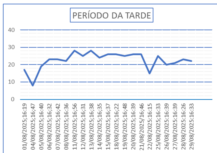
Gráfico 14 – Monitoramento de Pressão PCP -06.
