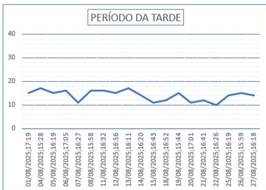
Gráfico 10 - Monitoramento de Pressão do PCP 04.
