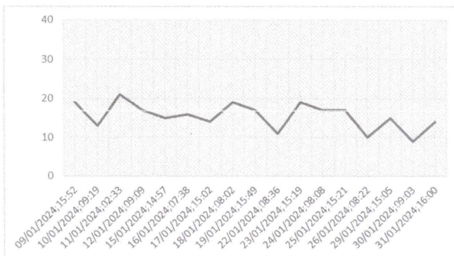
Gráfico 02 – Monitoramento de Pressão do PCP 01.
