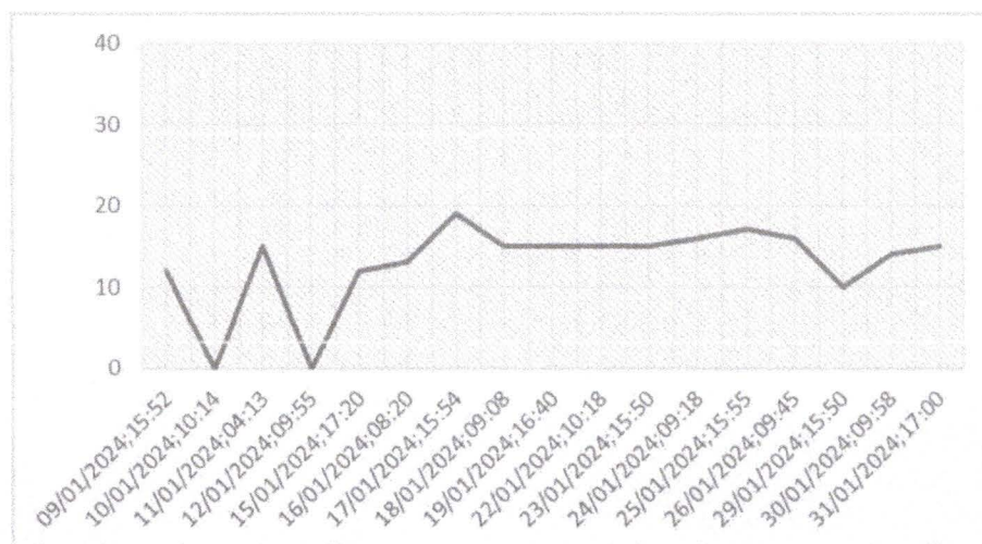
Gráfico 08 – Monitoramento de Pressão do PCP 07.
