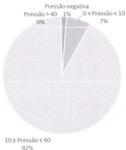
Gráfico 01 – Descrição do monitoramento de pressão.
